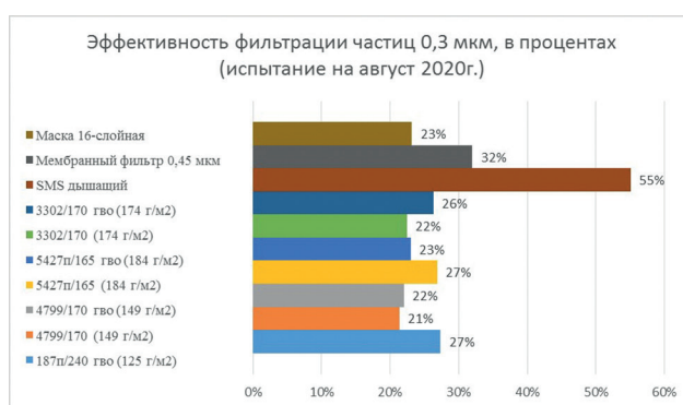
Диаграмма 5 - Анализ пор материалов на уровне 0,3 мкм 2 .
