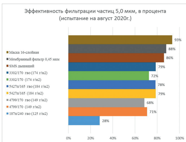
Диаграмма 7 - Анализ пор материалов на уровне 5,0 мкм 2 .
