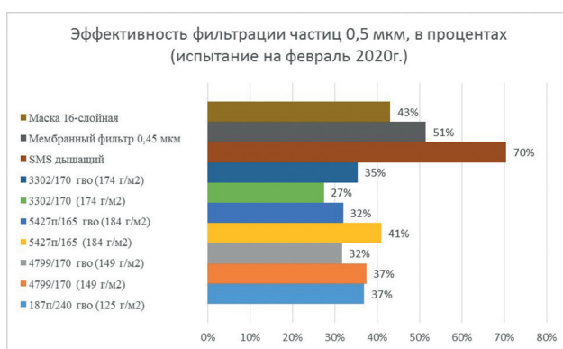
Диаграмма 3 - Анализ пор материалов на уровне 0.5 мкм 2 .
