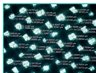
Рисунок 6 - Визуальное изображение структуры хлопчатобумажной ткани ГВО 4799-170 и его размер пор.
