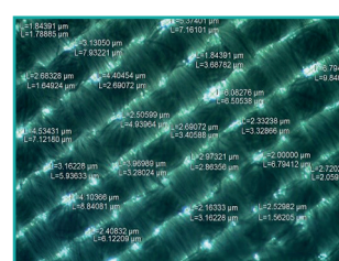
Рисунок 4 - Визуальное изображение структуры хлопчатобумажной ткани ГВО 5427-165 и его размер пор.
