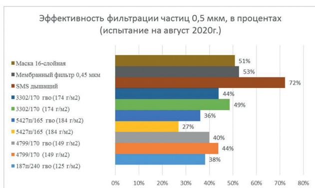
Диаграмма 6 - Анализ пор материалов на уровне 0,5 мкм 2 .
