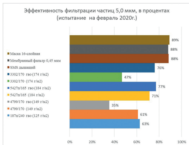
Диаграмма 4 - Анализ пор материалов на уровне 5.0 мкм 2 .
