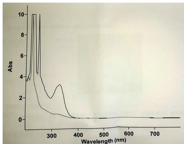
Рисунок 2 - Спектры поглощения левотироксина в стандартном образце (1) и нанопреparate (2) (растворитель - 10%-ный раствор NaOH, толщина кюветы - 10 мм).
