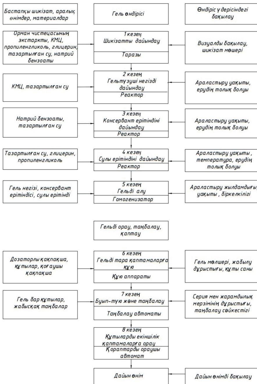
Технологиялық сызба 1 – Орман қайысқақшөп сығындысы бар гельдің алыну технологиясы
